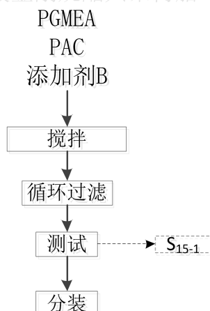
图 12 RDT500 248nm 厚膜光刻胶项目工艺流程图
