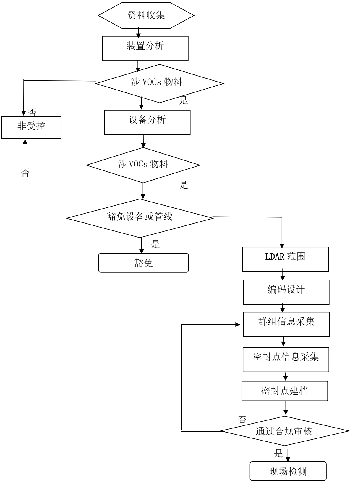
图 1.3.2-1 LDAR 项目建立流程图
