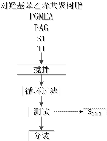
图 11 NRD6015-5 248nm 负性光刻胶项目工艺流程图
